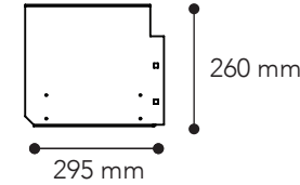
Istuintason kannatin
