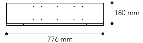
Hyllyn tausta 800
