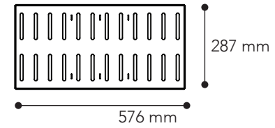
Hyllyn väljakaja
