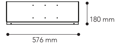
Hyllyn tausta 600
