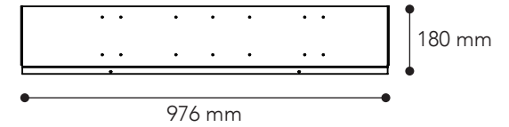
Hyllyn tausta 1000
