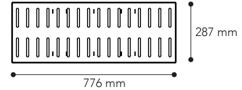
Hyllyn väljakaja
