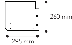
Istuintason kannatin
