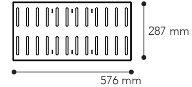
Hyllyn väljakaja
