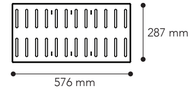
Hyllylevy 600
