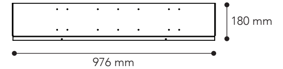
Hyllyn tausta 1000
